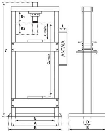
ΔΙΑΣΤΑΣΕΙΣ (mm)
